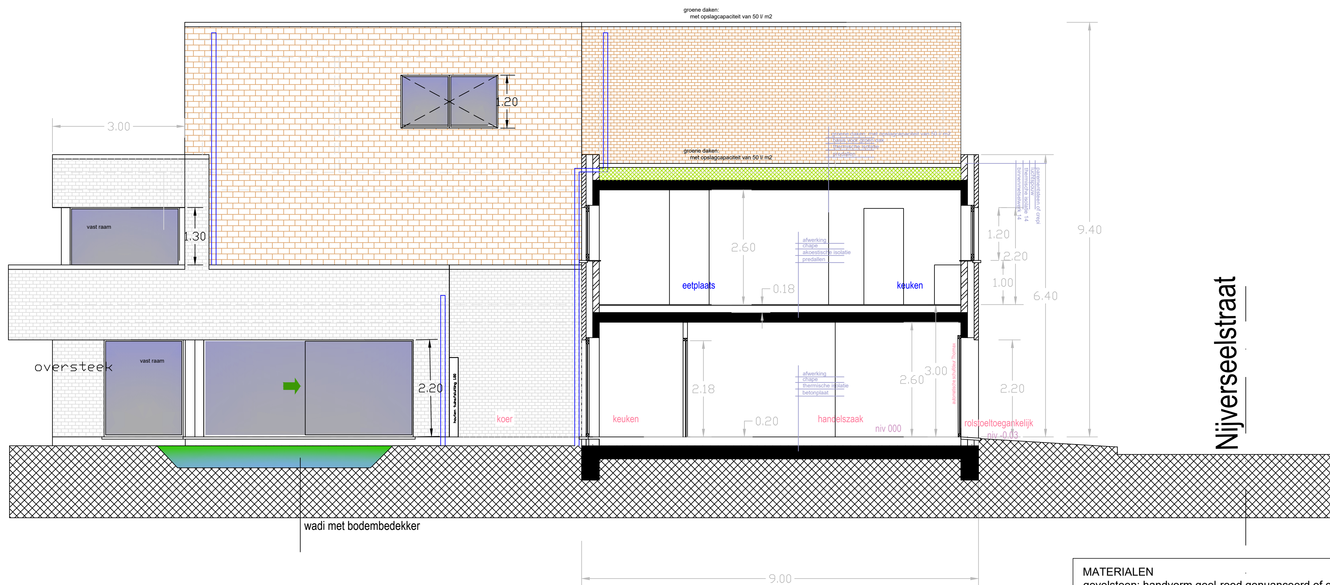
ACHTERGEVEL schaal 1/50
